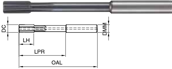
1678(止まり穴用) クーラント供給方式:センタースルー
