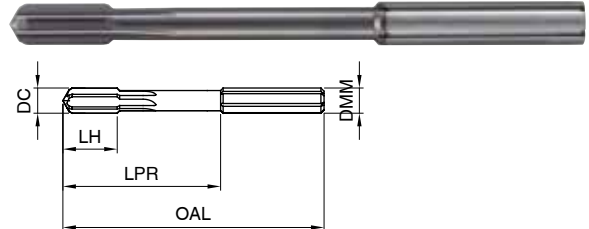
1679(貫通穴用) クーラント供給方式:シャンクスルー
